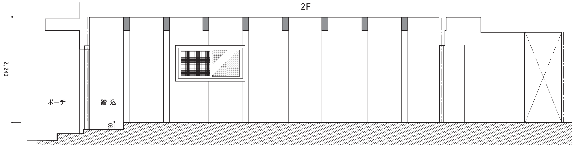
北側立面
