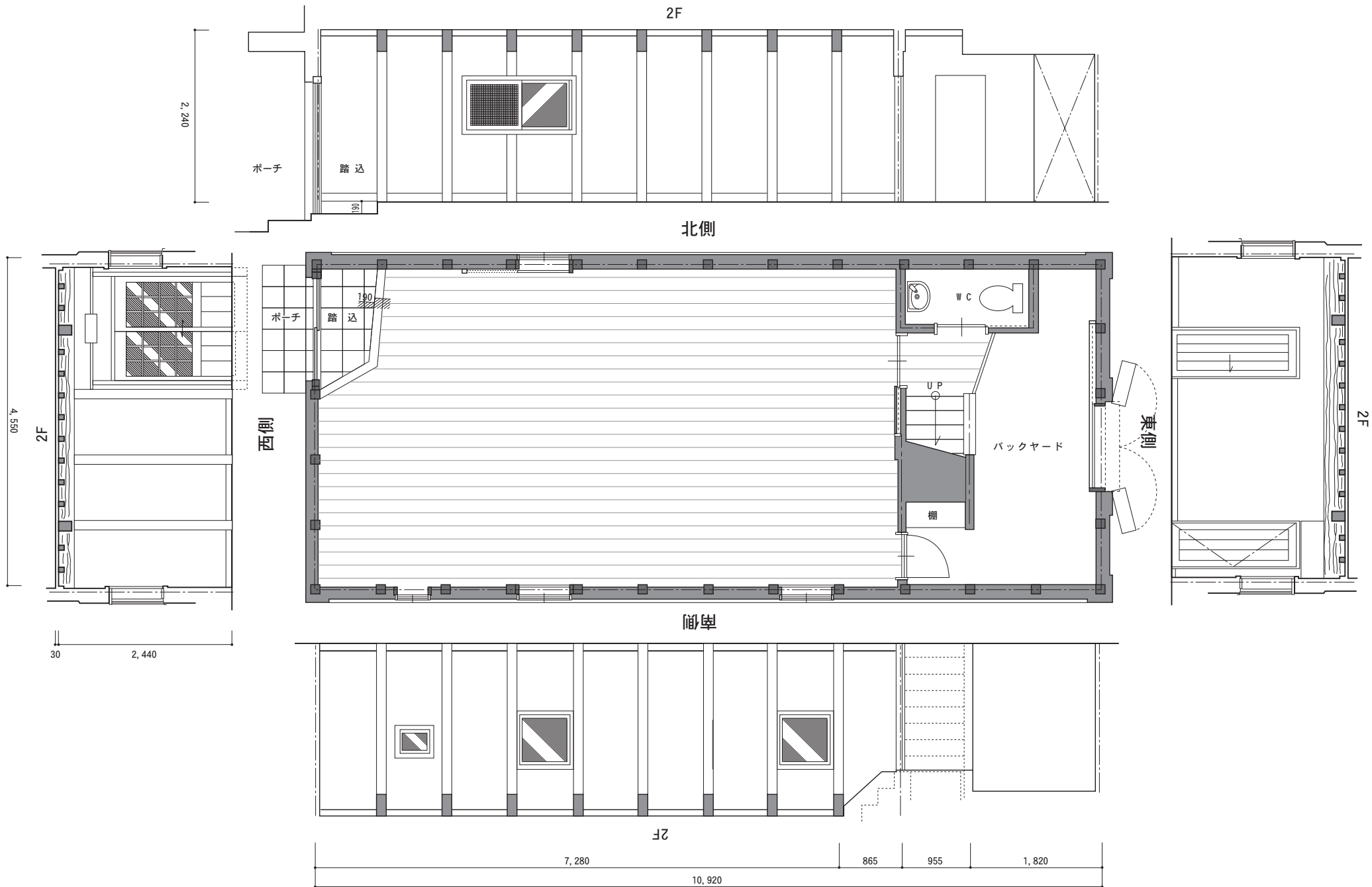
信濃ギャラリー 展開図
